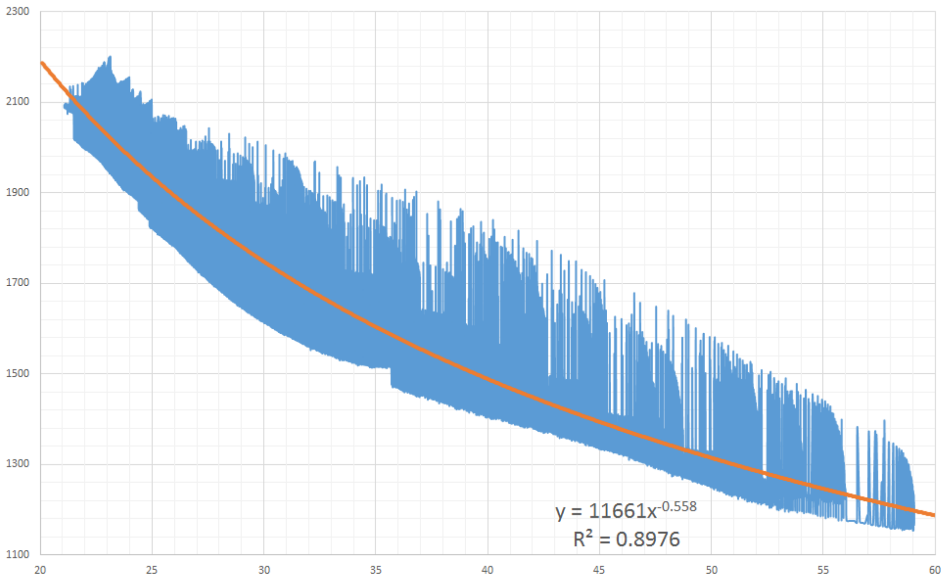
正极粘结剂粘度
